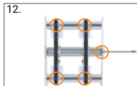
12. Riemenschwerte platzieren, Verbindungsschrauben anziehen und Motorrolle befestigen
