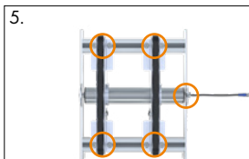
5. Position der Riemenschwerters anzeichnen, Verbindungsschrauben und Motorrolle lösen
