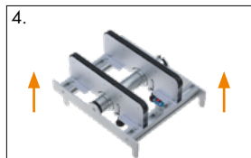
4. Hubeinheit herausheben
