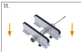
11. Riemenschwerters und Motorrolle platzieren
