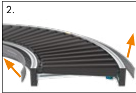
2. Abdeckprofile beidseitig ent- fernen
