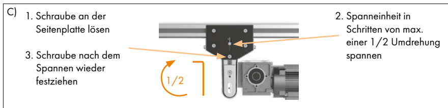
Gurt verläuft nach rechts, links spannen Gurt verläuft nach links, rechts spannen
