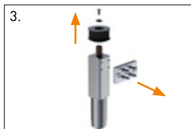
3. Zahnriemenscheibe und Motorplatte vom Motor entfernen
