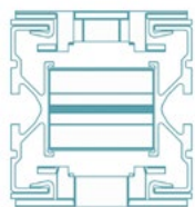
Larghezza telaio 87 mm
