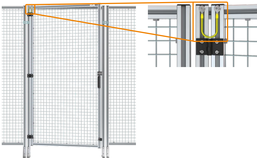
Illustration 1: Mise à la terre d'une porte simple
