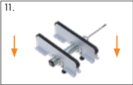
11. Colocar los soportes elevables y el rodillo motorizado
