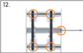
12. Colocar los soportes elevables, apretar los tornillos y fijar el rodillo motorizado
