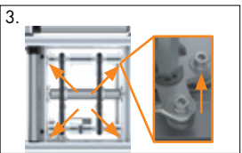
3. Retirar los 4 tornillos de conexión
