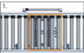
1. Retirar los rodillos en la zona del sistema de transferencia perpendicular
