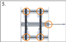
5. Marcar la posición de los soportes elevables, aflojar los tornillos y desconectar el rodillo motorizado
