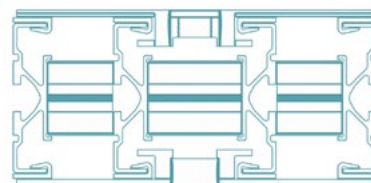
Šířka rámu 195 mm
