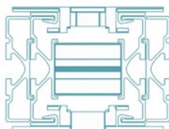
Šířka rámu 124 mm
