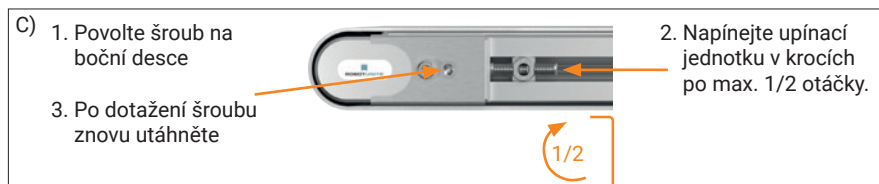
Seřízení pásového dopravníku
