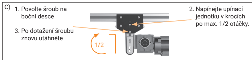
Seřízení pásového dopravníku
