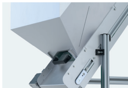
Vyprazdňovací otvor se zajišťovacím šoupátkem a ukazatelem stavu naplnění opticky
