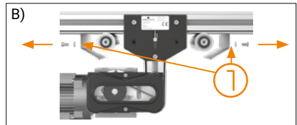
Einschnürtrommel entfernen
