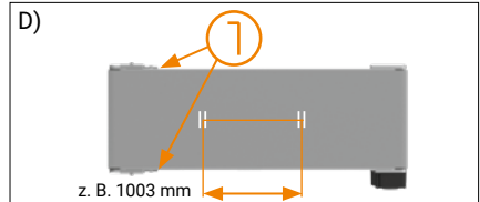
Spannen laut spezifischer Stückliste (z. B. 0,3 % = 1003 mm)
