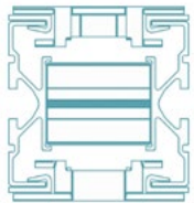
Rahmenbreite 87 mm
