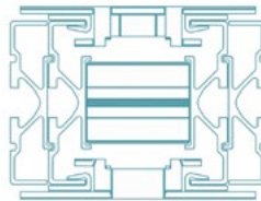
Rahmenbreite 124 mm
